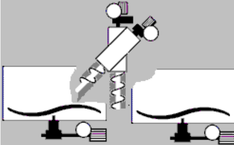
Abbildung 12: Doppelrondomat Obeneinbringer (Typ 41)
