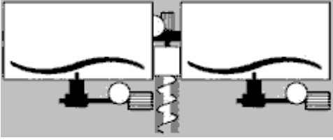
Abbildung 11: Doppelrondomat Unteneinbringer (Typ 40)
