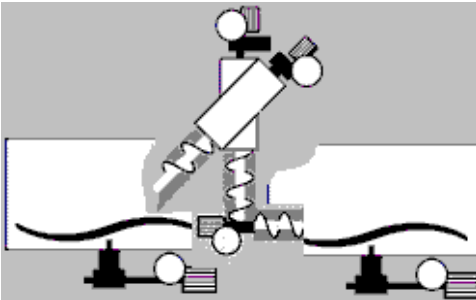
Abbildung 13: Doppelrondomat Obenhinteneinbringer (Typ 42)
