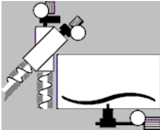
Abbildung 4: Rondomat Obeneinbringer (Typ 11)
