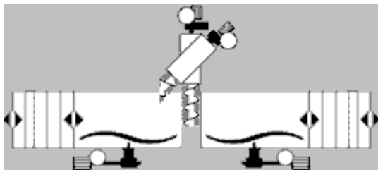
Abbildung 15: Biomat mit Anbaurondomat als Duplexanlage Obeneinbringer (Typ 51)
