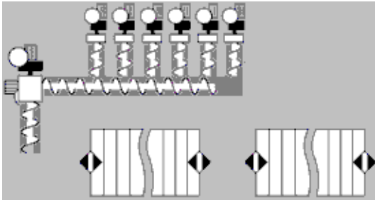
Abbildung 19: Biomat mit Duplexdosieraggregat als Duplexanlage Unteneinbringer (Typ 70)
