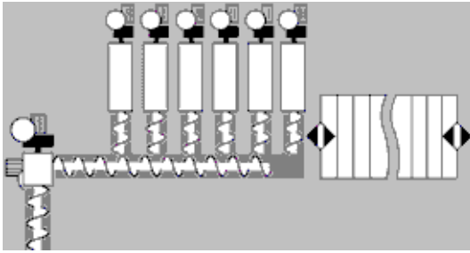
Abbildung 9: Biomat mit Duplexdosieraggregat Unteneinbringer (Typ 30)
