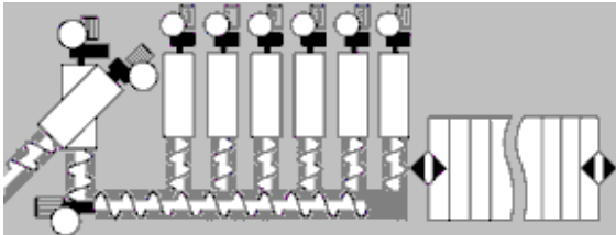
Abbildung 10: Biomat mit Duplexdosieraggregat Obeneinbringer (Typ 31)
