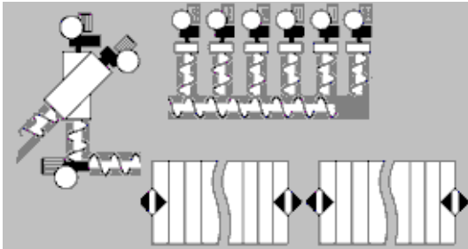
Abbildung 20: Biomat mit Duplexdosieraggregat als Duplexanlage Obeneinbringer (Typ 72)
