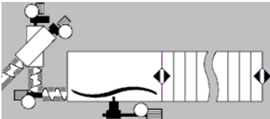
Abbildung 8: Biomat mit Anbaurondomat Obenhinteneinbringer (Typ 22)
