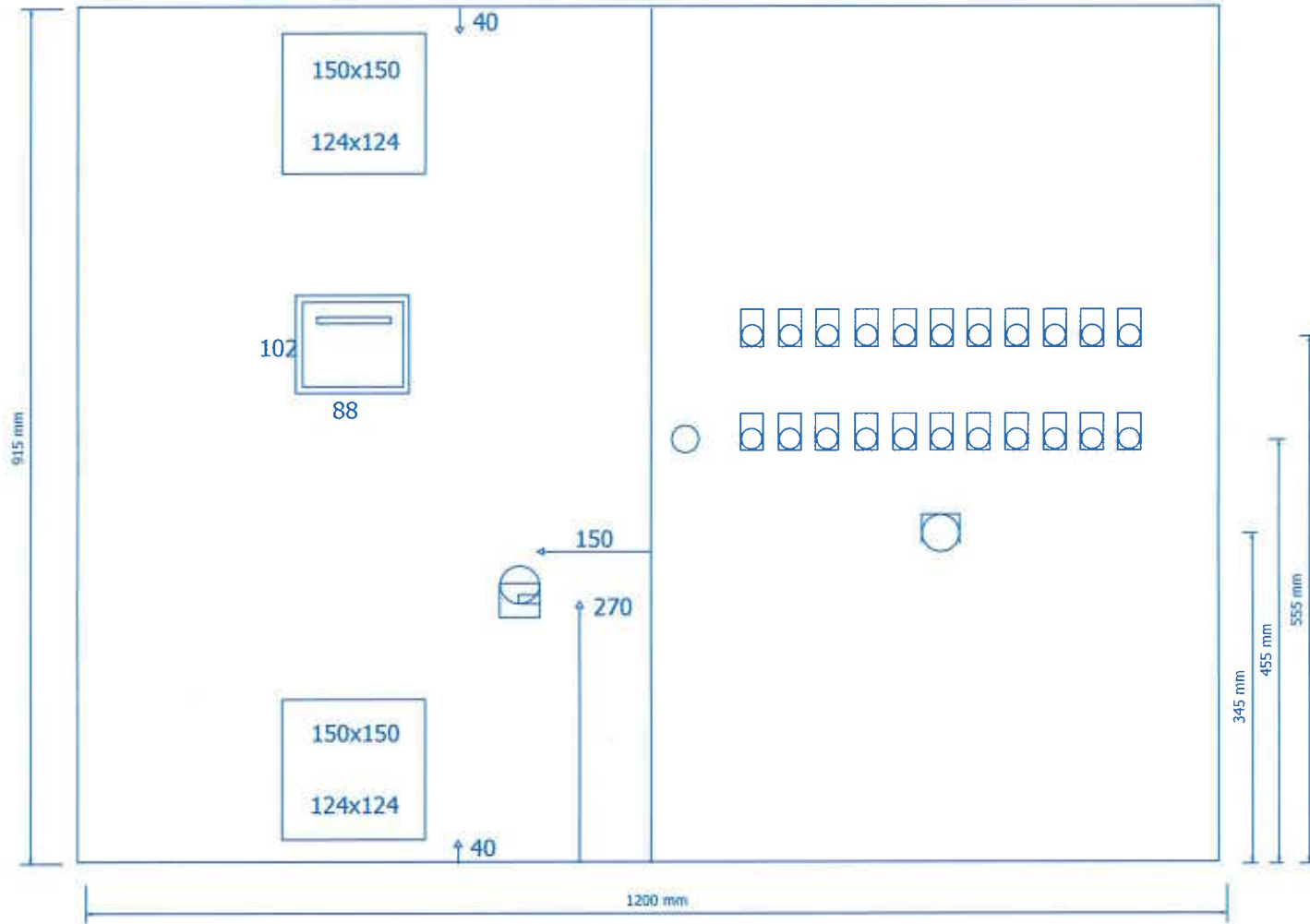
Schalschrank Häwa 3331-1291-30-07 1200x915x300
