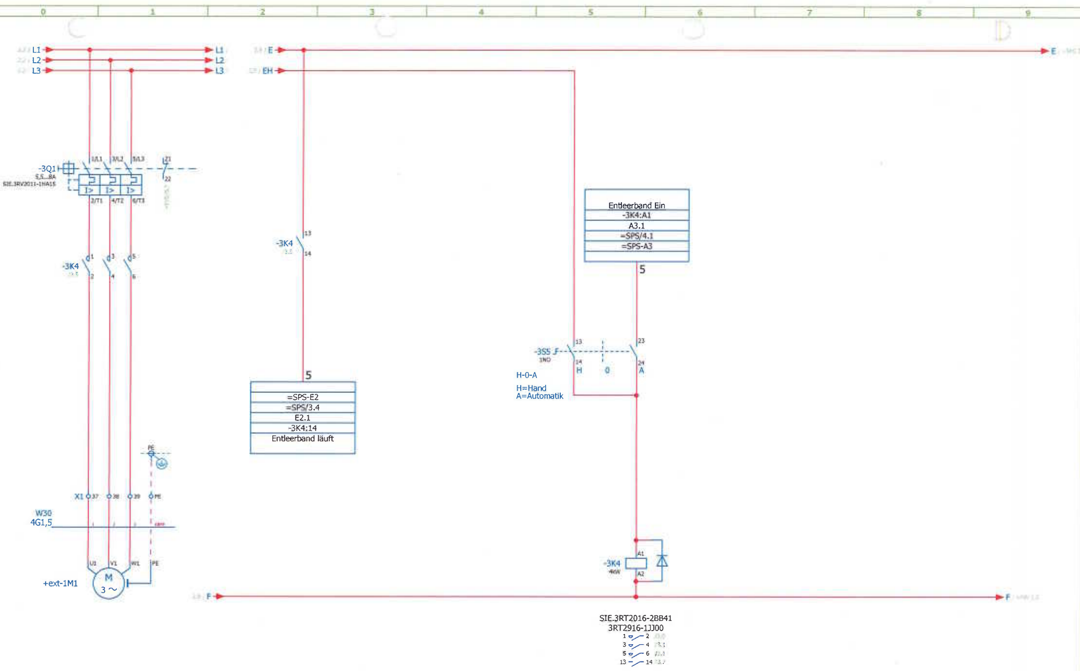
Entleerband 3kW
