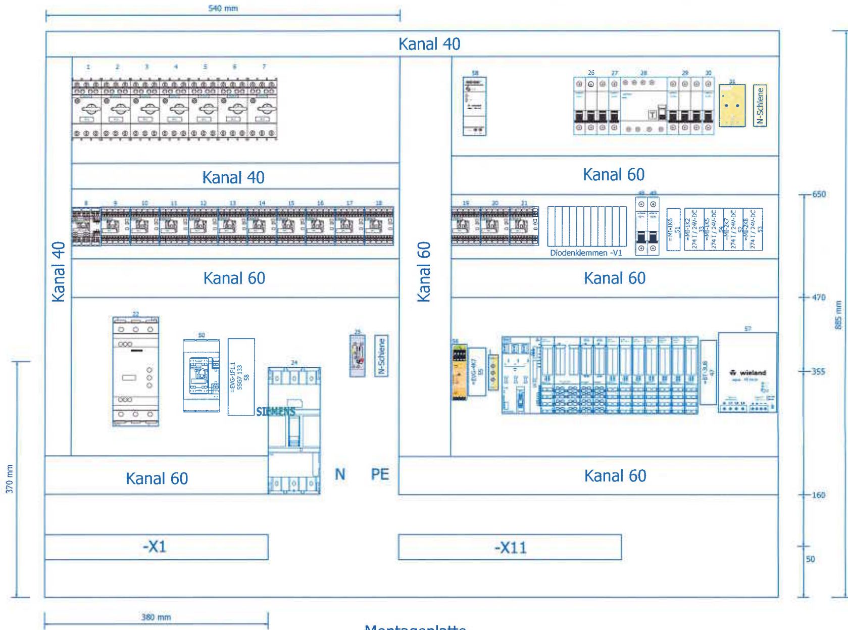
Montageplatte 1128x885
