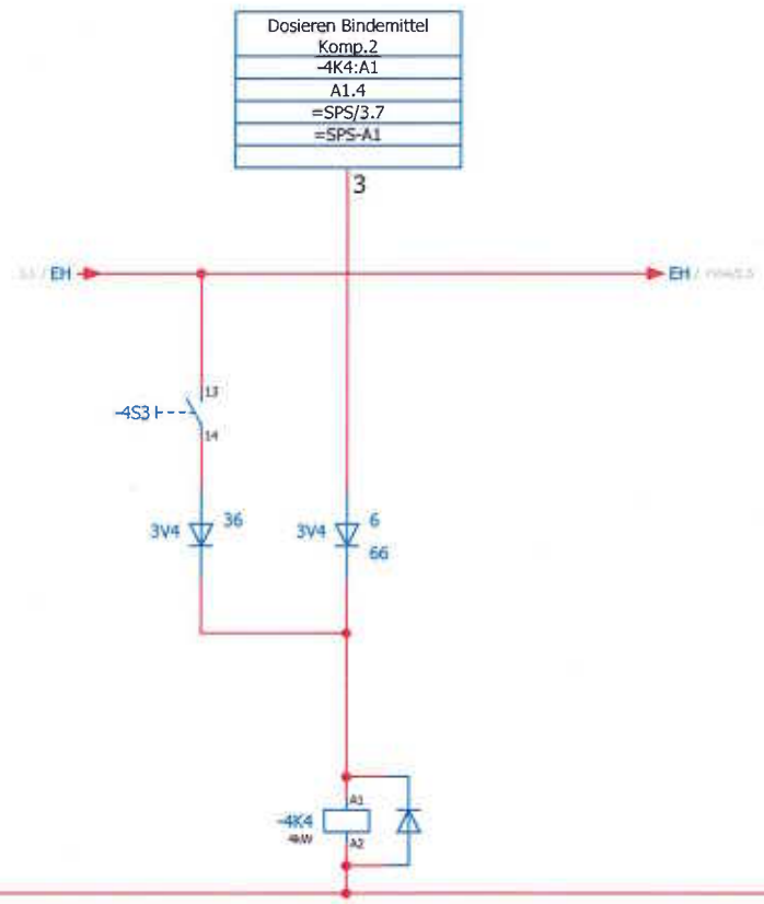
SIE.3RT2016-2BB41 3RT2916-1JJ00 1 2 / 5,0 3 4 / 4,1 5 6 / 4,1 13 14 / 5,0
